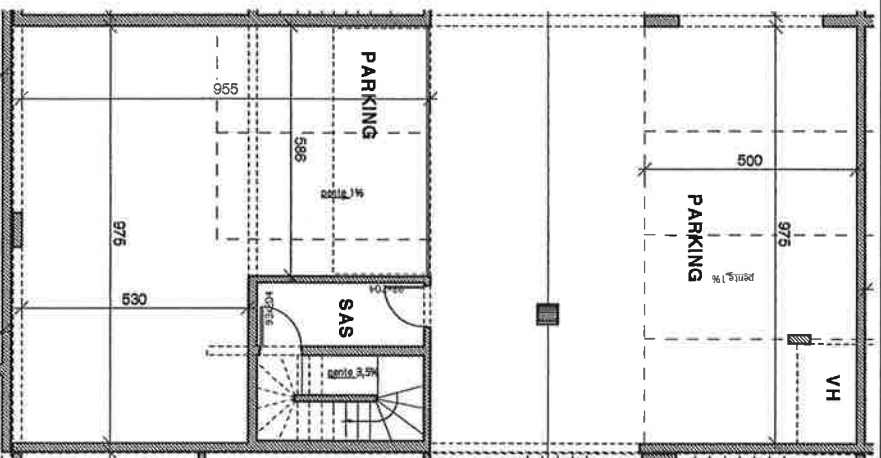
SOUS-SOL
